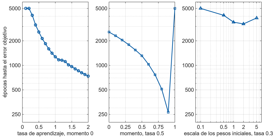
Figura 2: Épocas hasta el error objetivo sobre la XOR de dos entradas al variar la tasa de aprendizaje, el momento y la escala de los pesos iniciales, cuatro neuronas ocultas y promedio de cinco semillas. Un valor de 5000 indica que no se alcanzó el objetivo. Escala logarítmica en el eje vertical, y el tercer panel usa tasa 0.3
