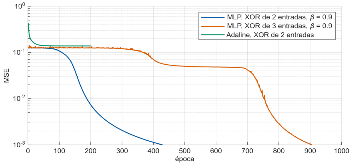
Figura 1: Curvas de error de entrenamiento sobre la XOR de dos y tres entradas con una de las cinco semillas, en escala logarítmica. El MLP con cuatro neuronas ocultas y momento 0.9 llega al error objetivo en ambos casos, y el Adaline se estanca cerca de 0.139, apenas por encima del piso de 0.125 de la mejor función lineal
